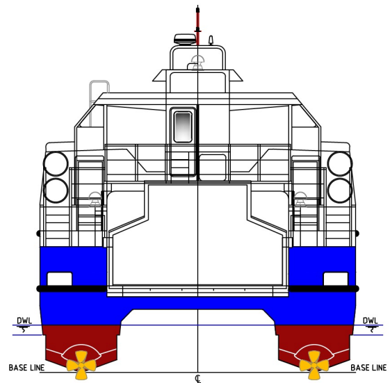
TAMPAK BELAKANG
