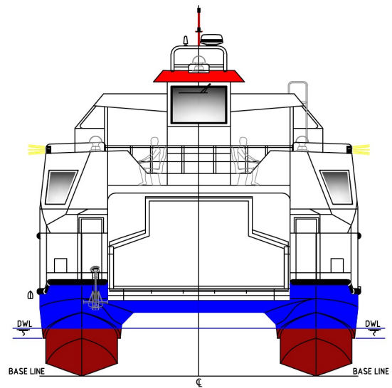
TAMPAK DEPAN
