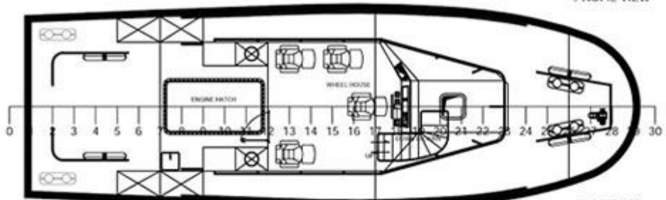
MAINDECK
